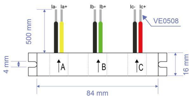
底视图
